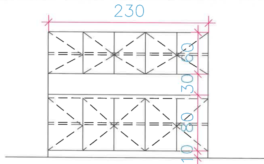
Elevation B-B
