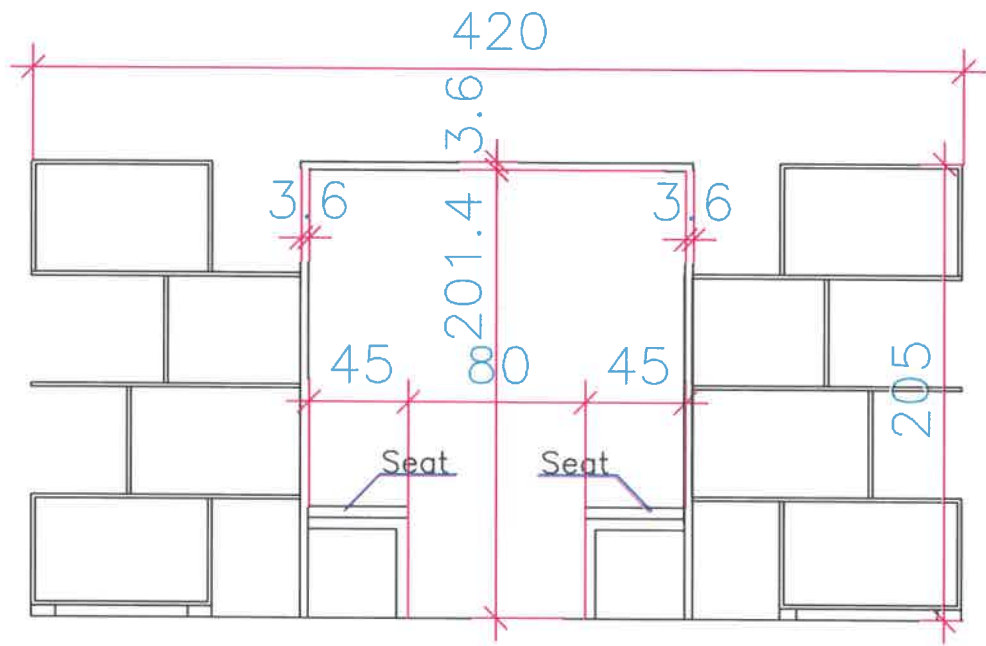
Elevation A-A
